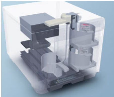
Tres depósitos para 50 soportes hacen posible producir hasta 100 soportes en un ciclo de trabajo de forma completamente automática.
